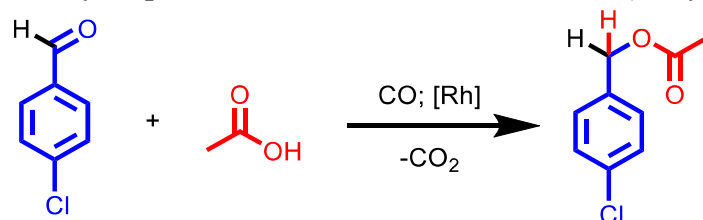
Рисунок 3. Восстановительная этерификация п-хлорбензальдегида уксусной кислотой
