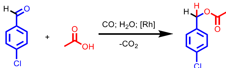
Рисунок 4. Восстановительная этерификация п-хлорбензальдегида уксусной кислотой в присутствии воды
