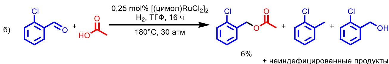
Рисунок 15. Проведение реакции этерификации в присутствии [(\text{цимол})\text{RuCl}_2]_2 в качестве катализатора; а – с использованием CO, синтез-газа и \text{H}_2 в качестве восстановителя, б – с использованием \text{H}_2 в качестве восстановителя
