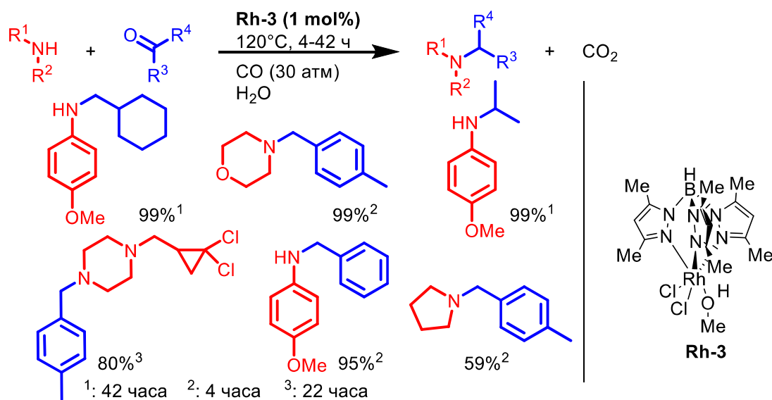
Рисунок 14. Серия реакций восстановительного аминирования
